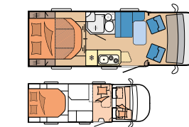
L: 6.979 mm · B: 2.230 mm H: 2.820 mm · G: 3.500 kg
